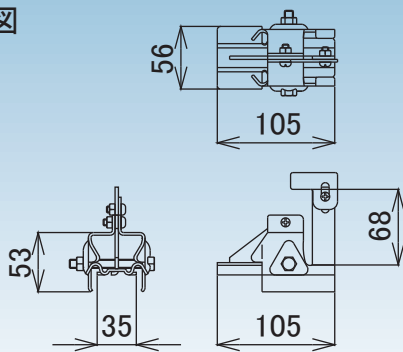
D-328 スノーストップ三晃式 A型
