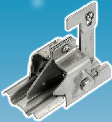
D-328 スノーストップ三晃式 A型
