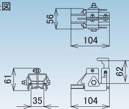
D-329 スノーストップ三晃式 B型
